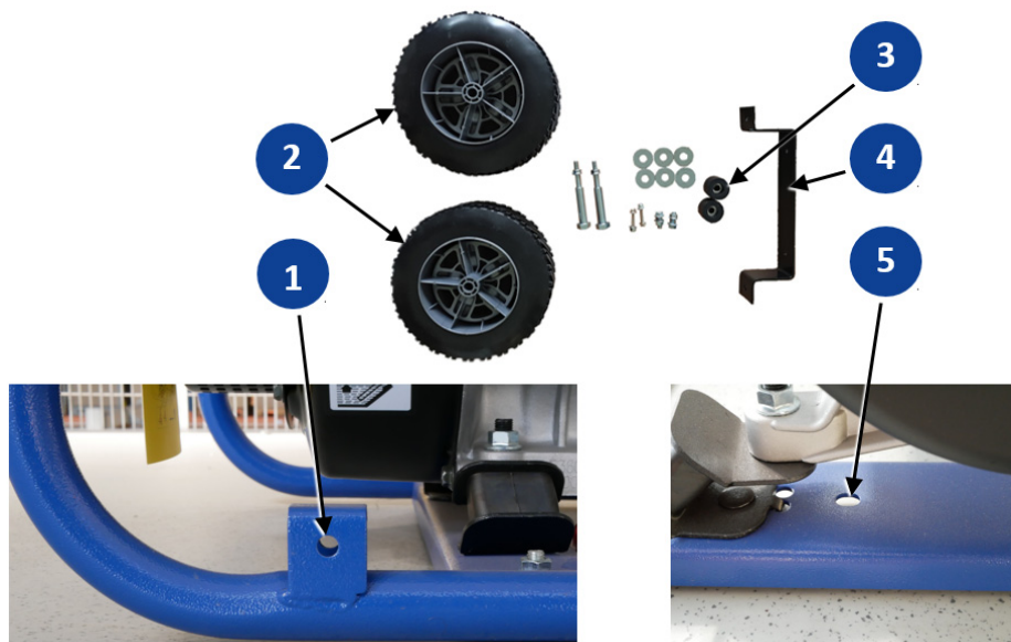
Fig. 7-1 Komponenter hjulsett
