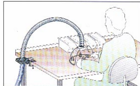
Flexibel arbetsplats. Lätt att byta placering av utsuget.
